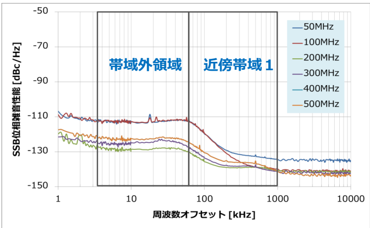
例）MS2830A+低位相雑音（opt.066） 位相雑音性能グラフ meas.
