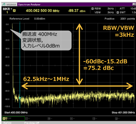
スプリアス領域 画面例 (近傍領域1)
